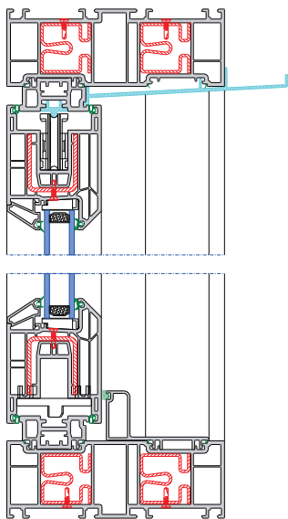
Sección vertical Elevadora
